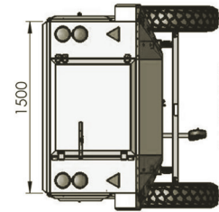
HECKANSICHT
